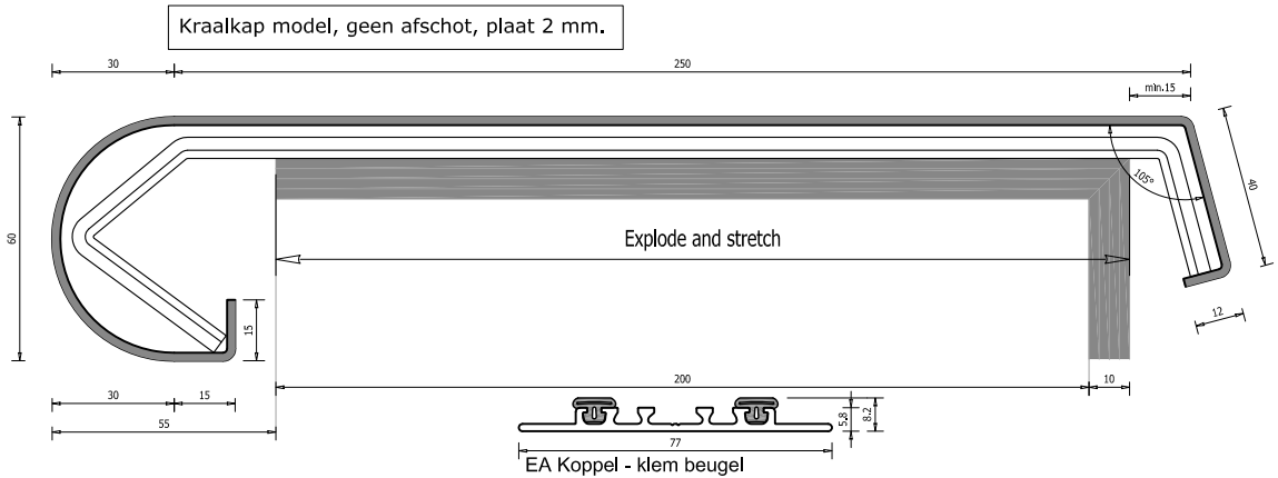
EA Map-KK-2pl-0afs-60-40 maatvoering
