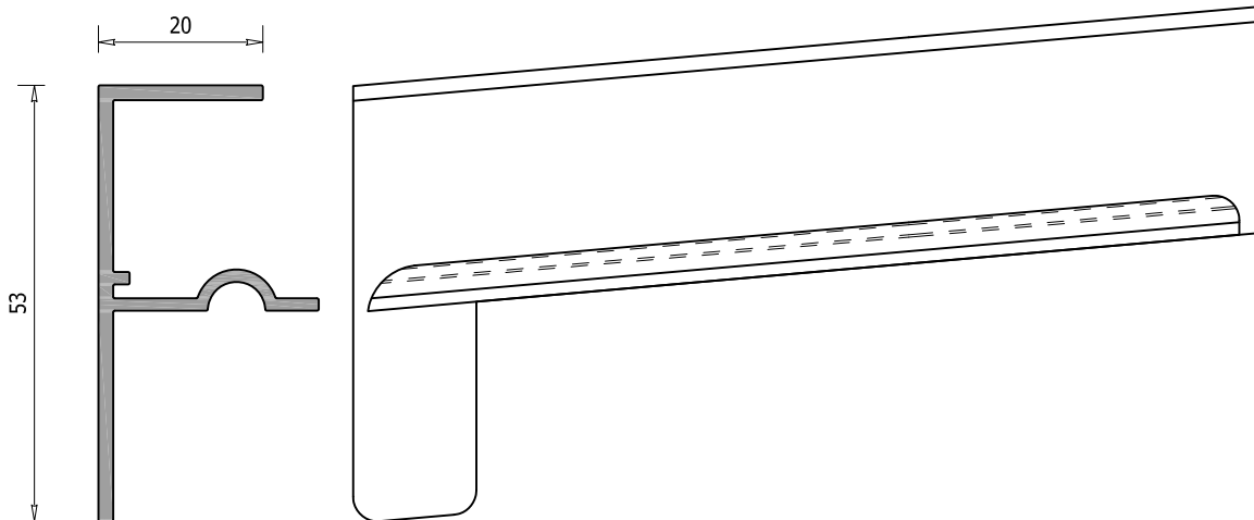
EA Kopschot type 6 voor waterslagprofiel 5°
