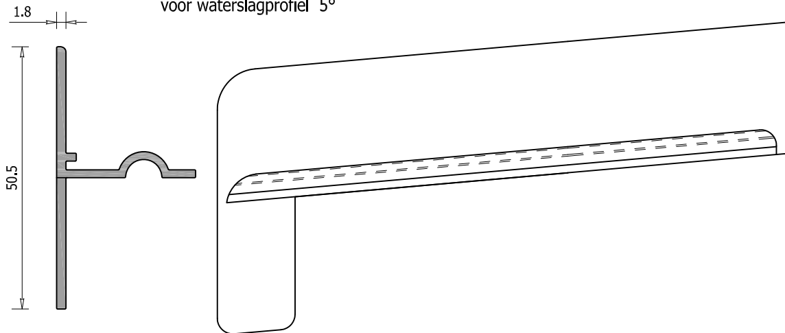
EA Kopschot type 4 voor waterslagprofiel 5°
