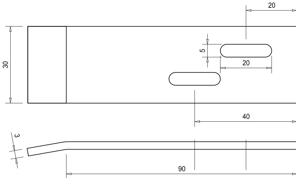
EA standaard anker 90 mm.
